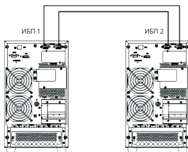
Рис. 2-3: 2 параллельных ИБП
