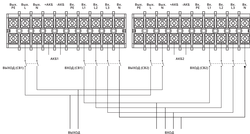
Рис. 2-2: Схема параллельного подключения
