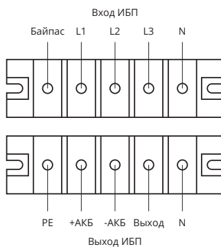
Рис 2- 1: Схема подключения клеммного блока
