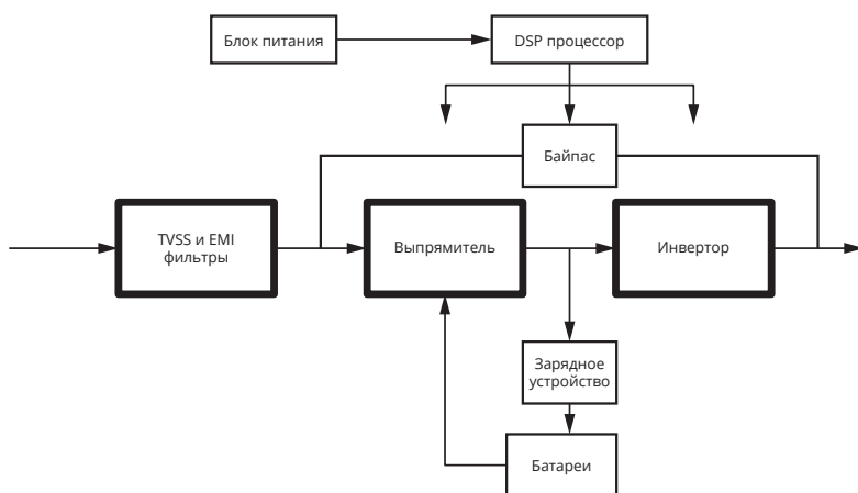
Рис 1-3: Система ИБП
