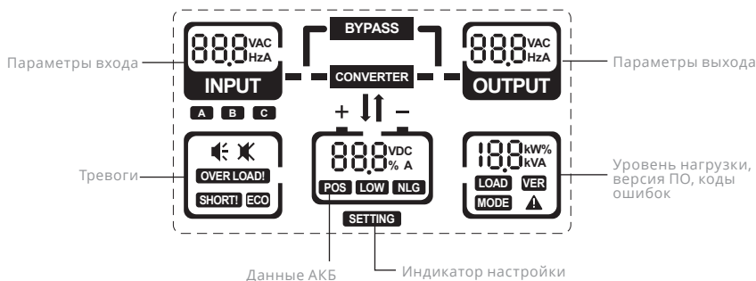
Рис. 3-2: Меню ЖК-дисплея
