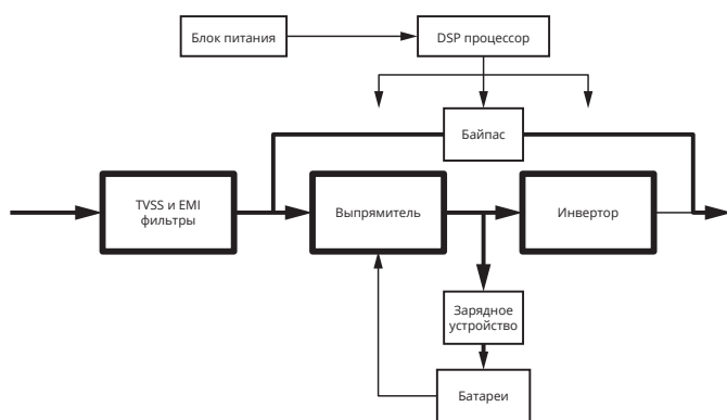
Рис. 1-7: Эко-режим
