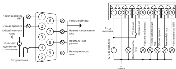
Рис. 5-2: Подключение к внешнему источнику питания
