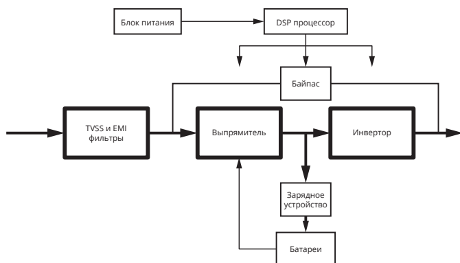
Рис 1-4: Нормальный режим
