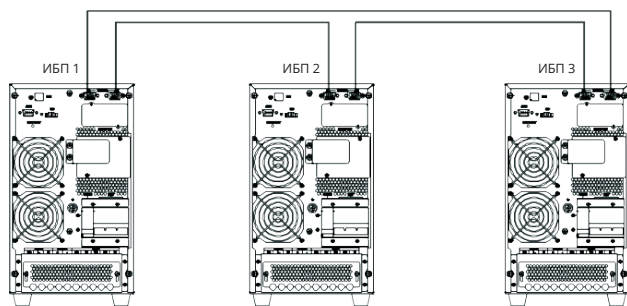
Рис. 2-4: 3 параллельных ИБП
