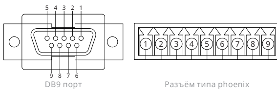
Рис. 5-1: Сухие контакты
