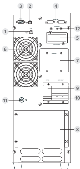
Рис. 1-2: Вид сзади
